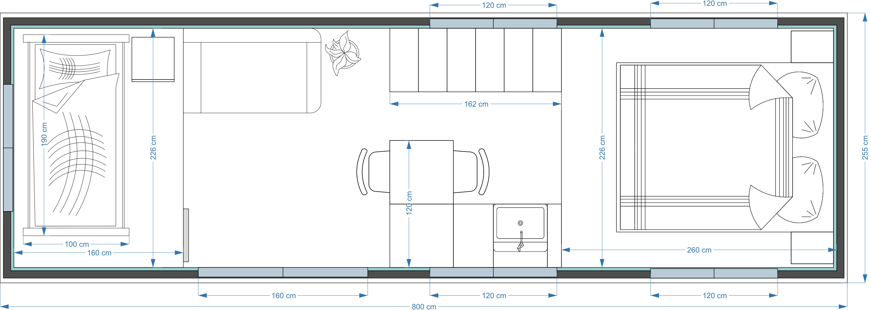
Loft Plan
