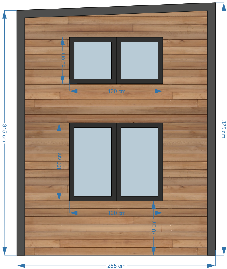
Sol cephe
