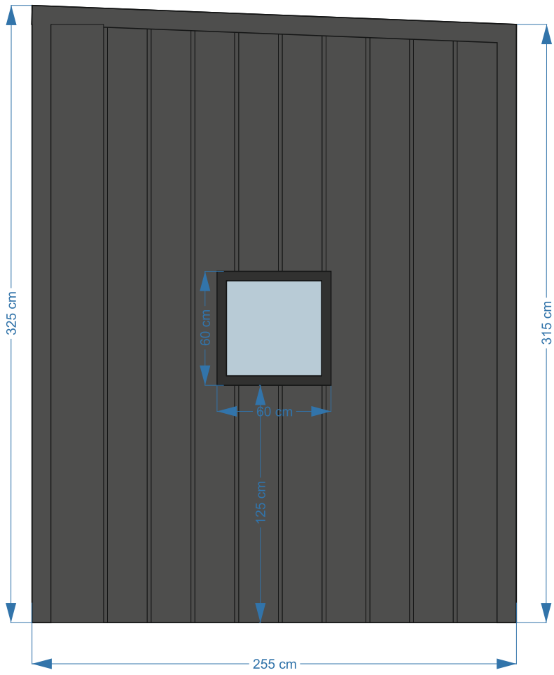
Sağ cephe
